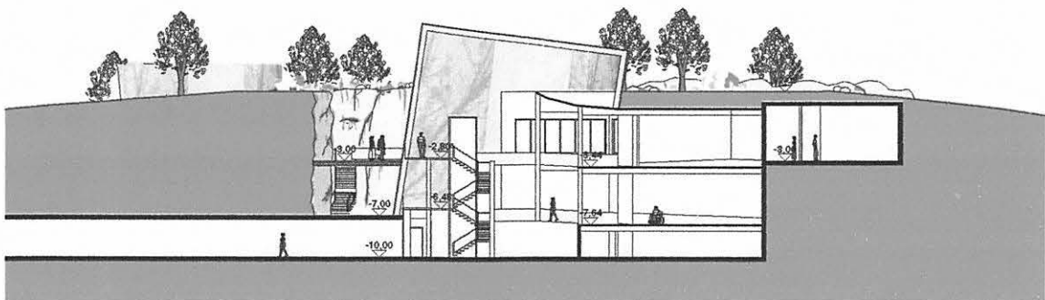
Schnitt 2
