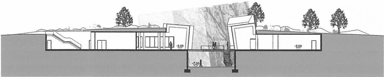
Schnitt 1
